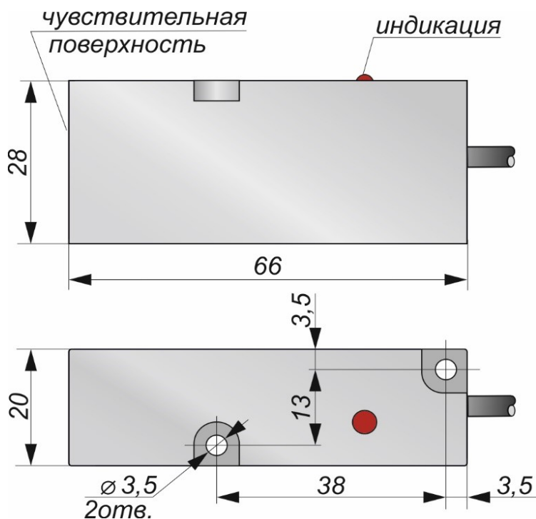
Габаритный чертеж
