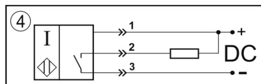
Нормально-разомкнутый контакт
