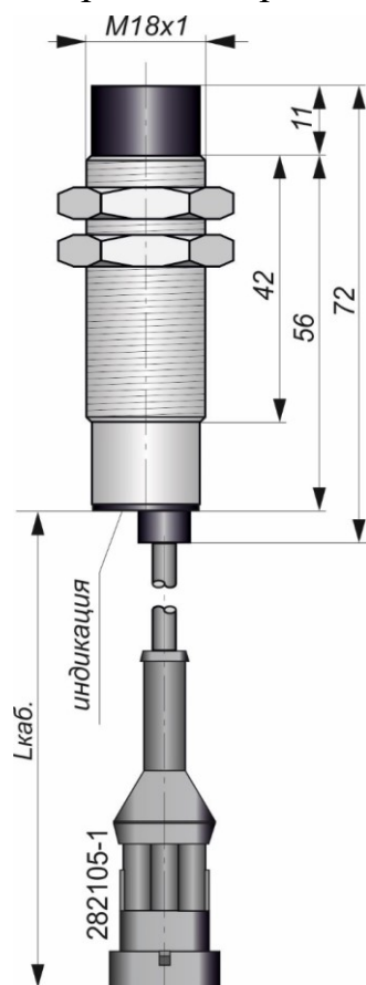
Габаритный чертеж
