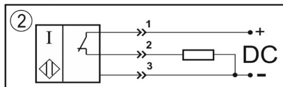
Нормально-замкнутый контакт
