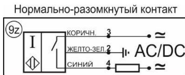
Схема соединения
