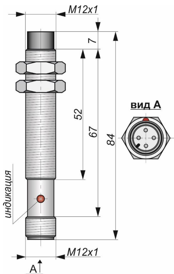
Габаритный чертеж
