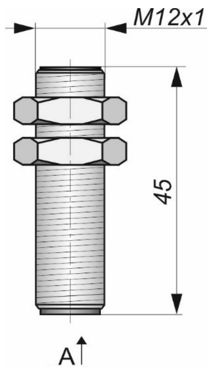
Габаритный чертеж
