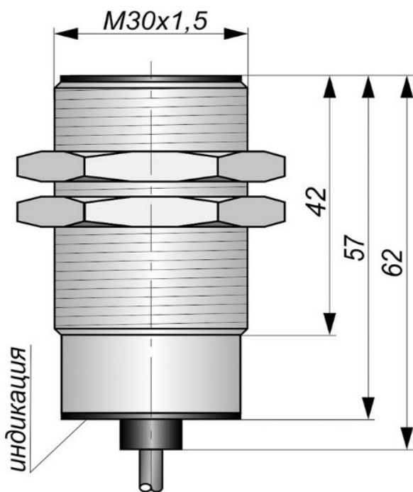
Габаритный чертеж
