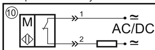
Схема подключения
