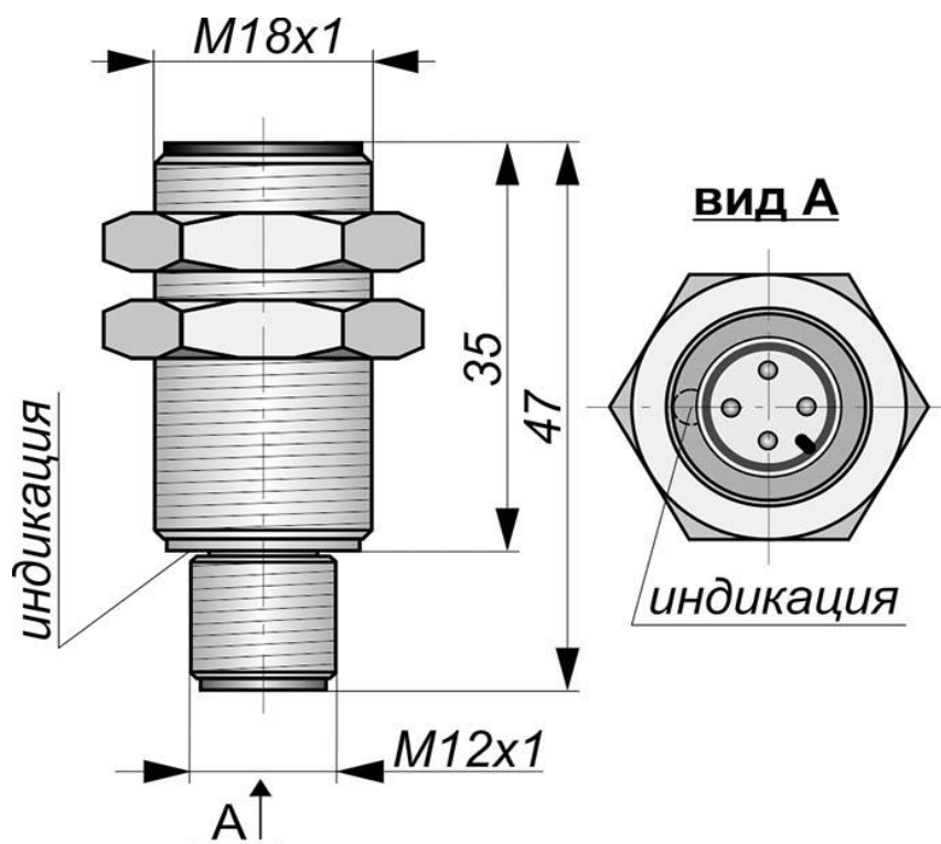
Габаритный чертеж
