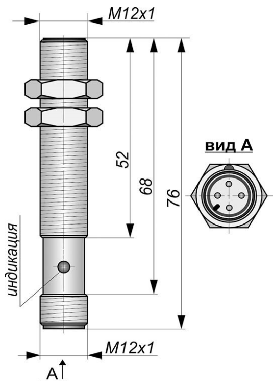
Габаритный чертеж
