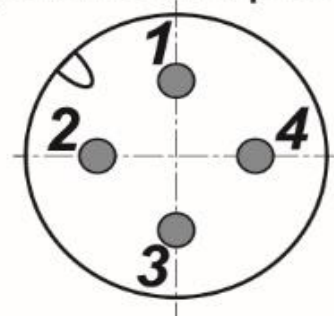
Цоколевка разъема
