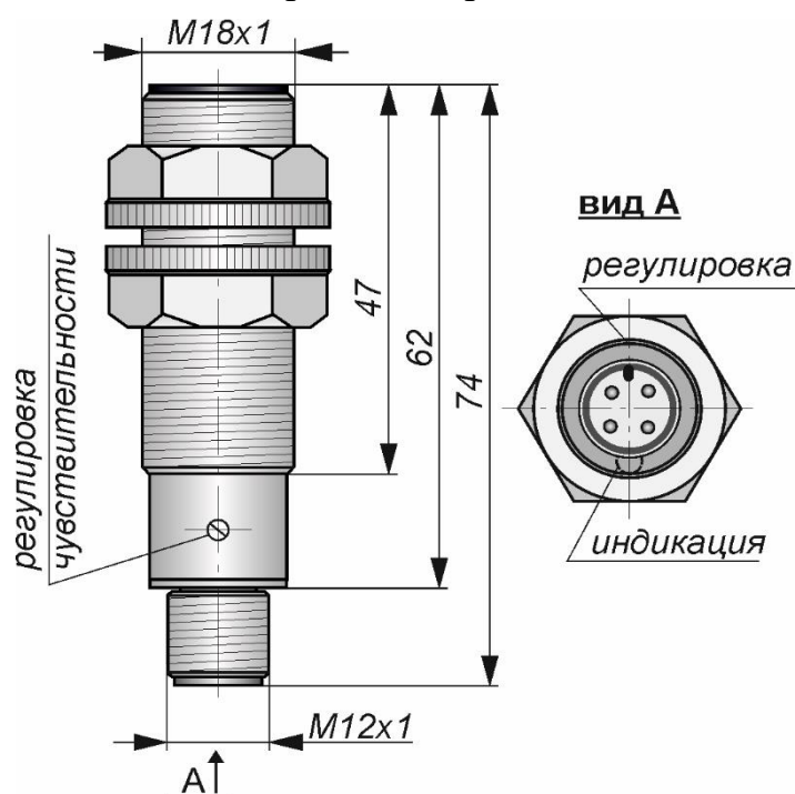
Габаритный чертеж
