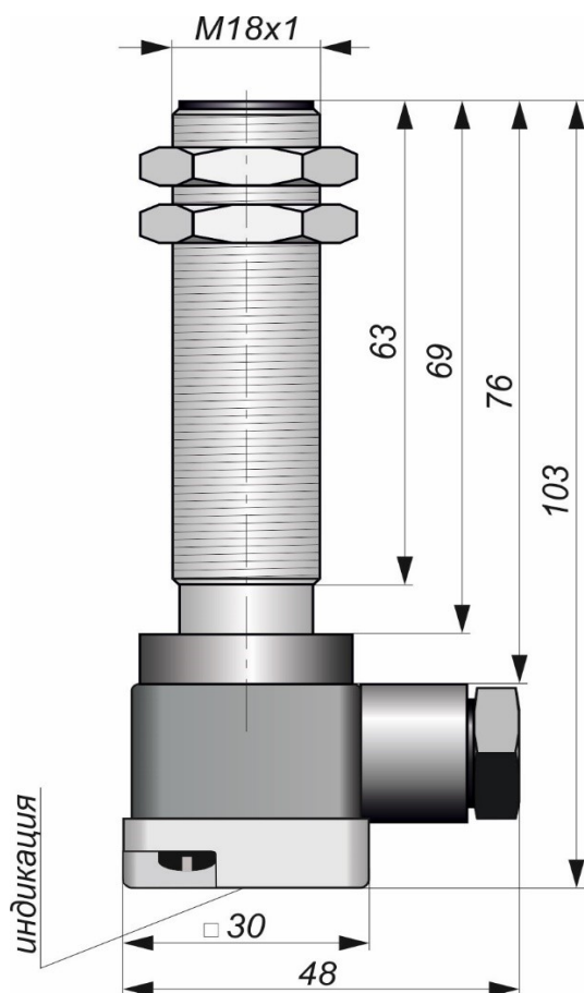
Габаритный чертеж
