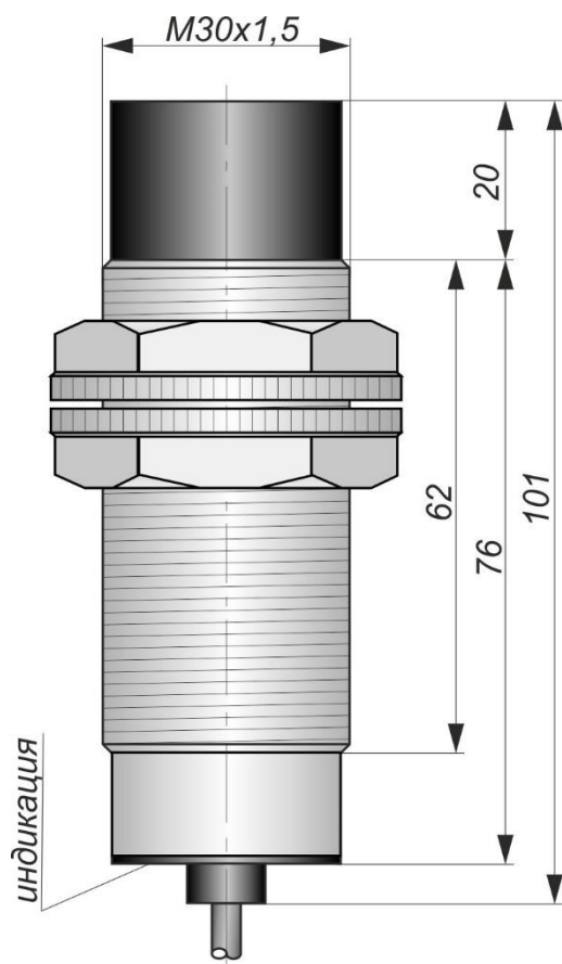
Габаритный чертеж
