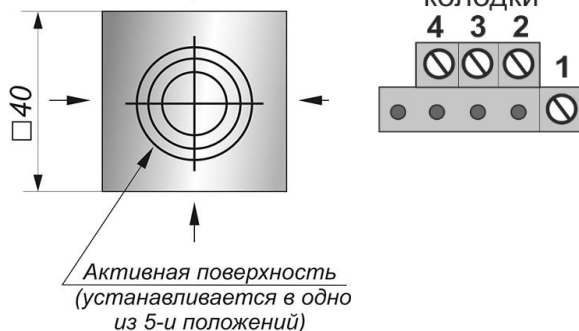
Цоколевка клеммной колодки
