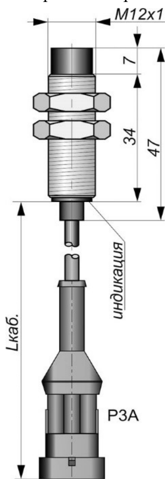
Габаритный чертеж
