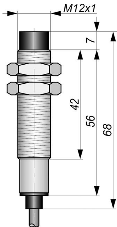
Габаритный чертеж
