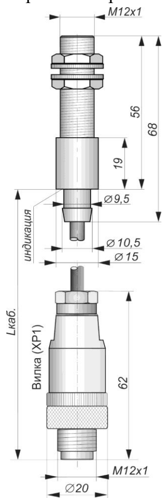
Габаритный чертеж
