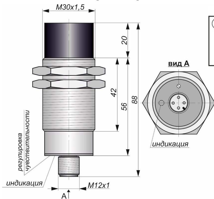
Габаритный чертеж
