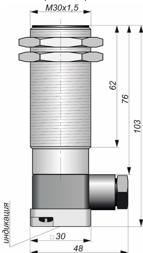
Габаритный чертеж
