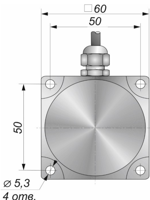
Габаритный чертеж
