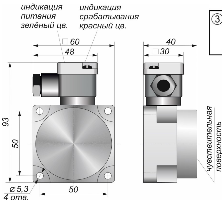
Габаритный чертеж
