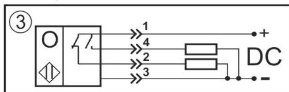
Цоколевка разъема
