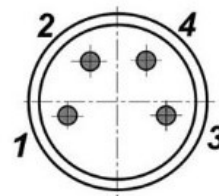
Цоколевка разъема
