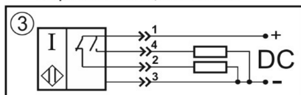
Переключающий контакт
