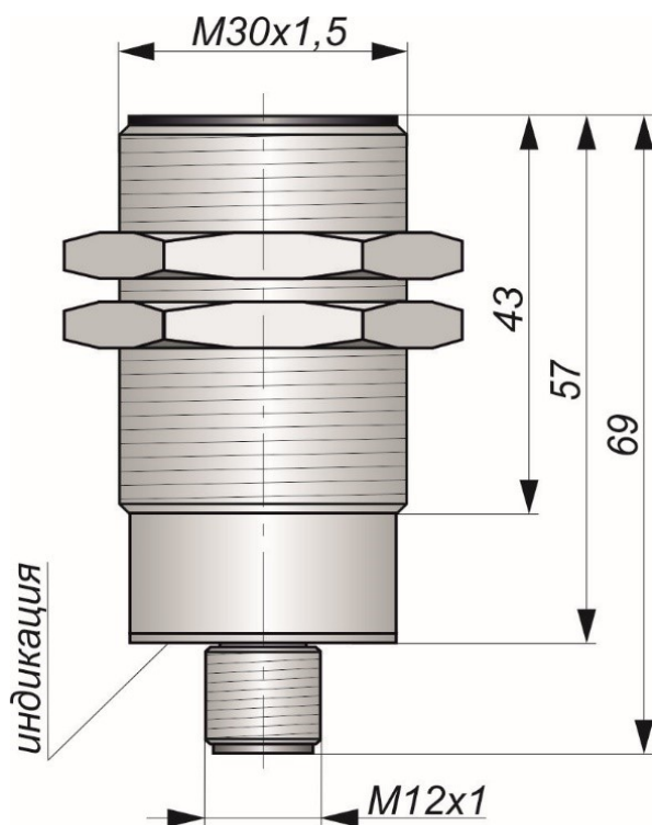
Габаритный чертеж
