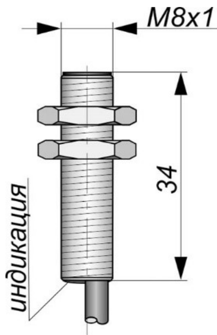
Габаритный чертеж
