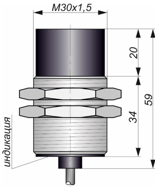
Габаритный чертеж
