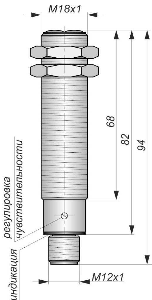
Габаритный чертеж
