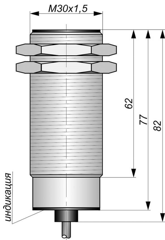
Габаритный чертеж
