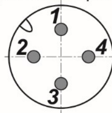
Цоколевка разъема
