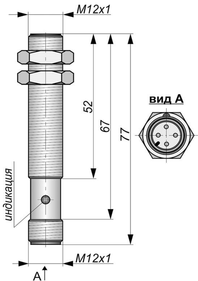
Габаритный чертеж
