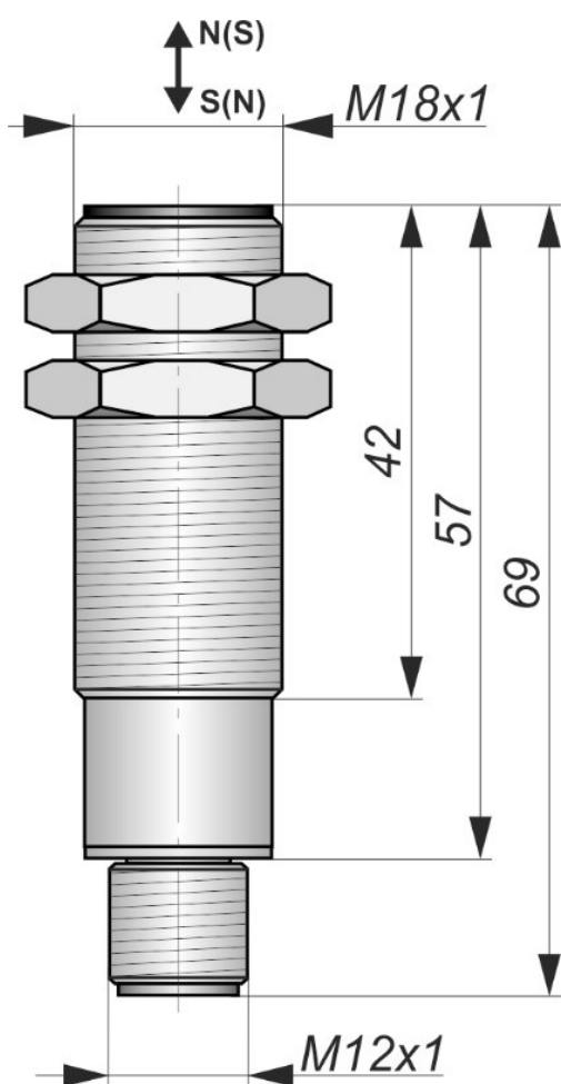
Габаритный чертеж
