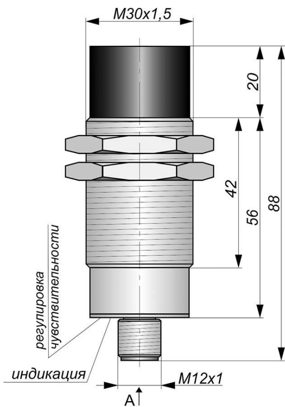
Габаритный чертеж
