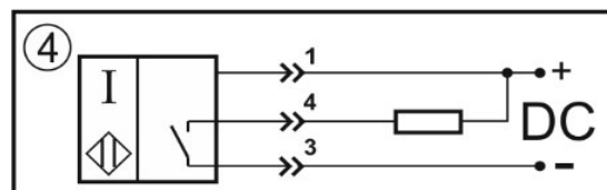
Цоколевка разъема
