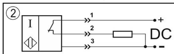
Нормально-замкнутый контакт
