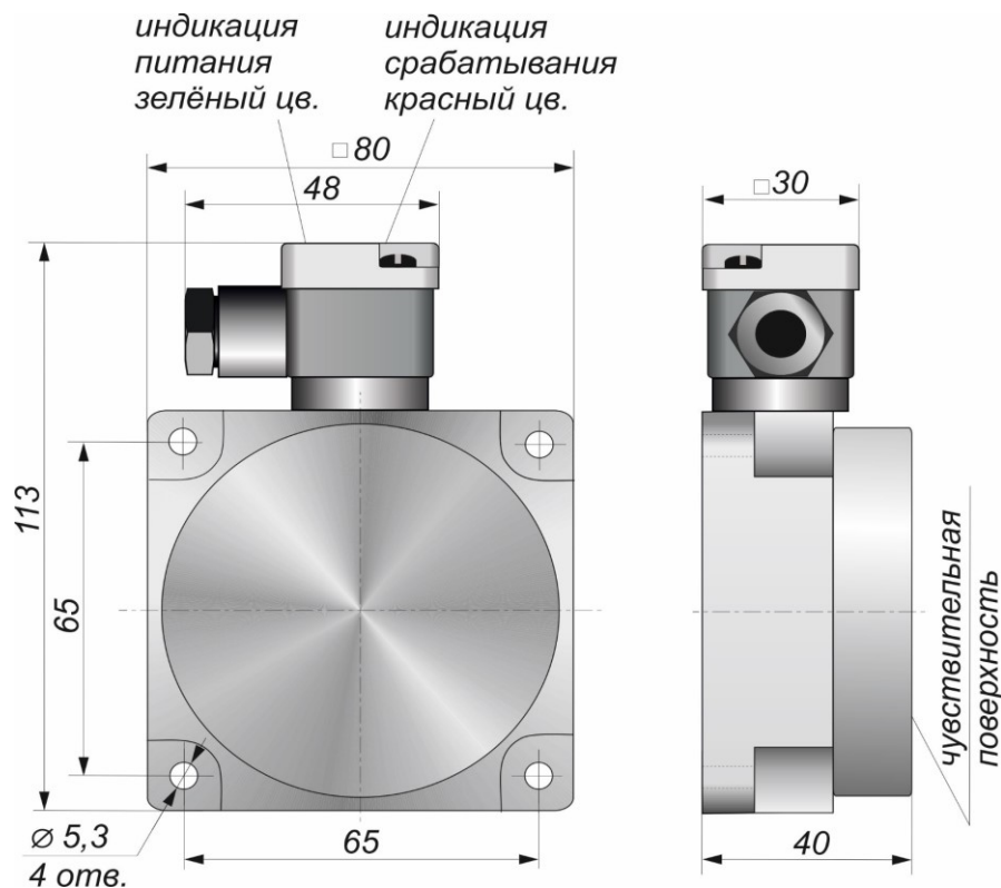
Габаритный чертеж
