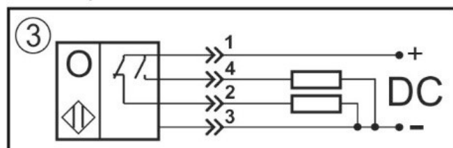
Схема соединения Переключающий контакт
