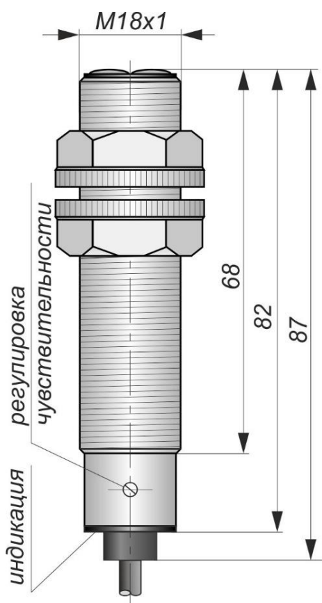
Габаритный чертеж
