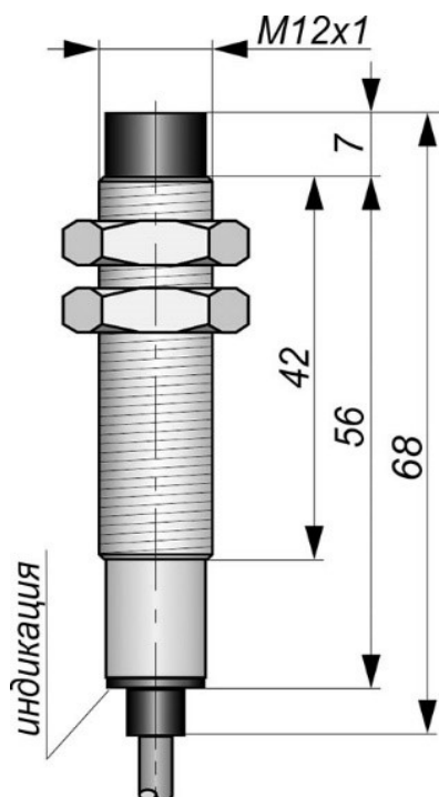
Габаритный чертеж
