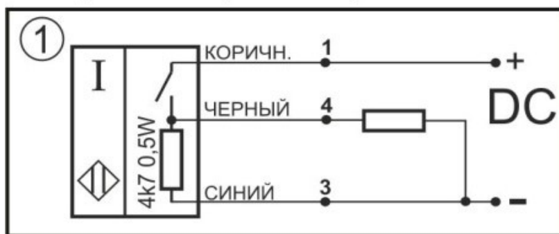
Нормально-разомкнутый контакт
