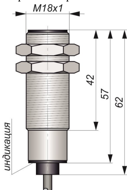
Габаритный чертеж
