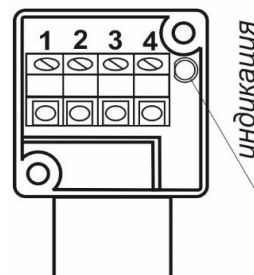
Цолевка клеммной колодки
