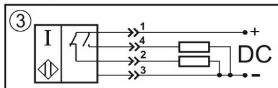
Переключающий контакт
