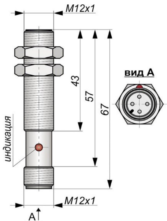
Габаритный чертеж
