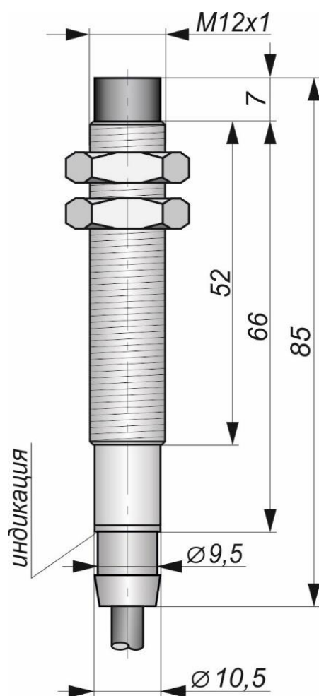
Габаритный чертеж
