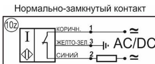
Схема соединения
