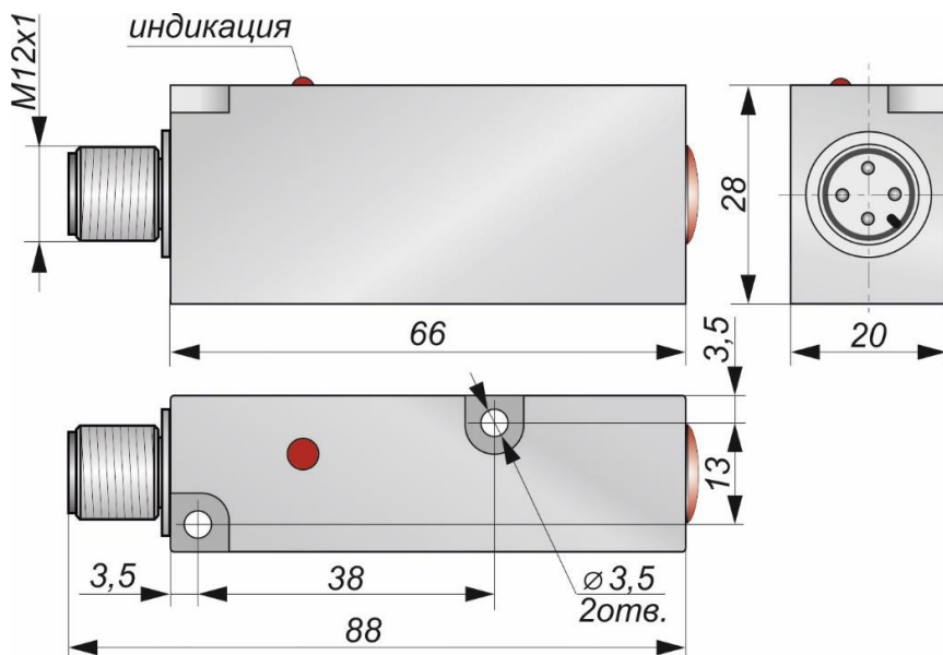
Габаритный чертеж
