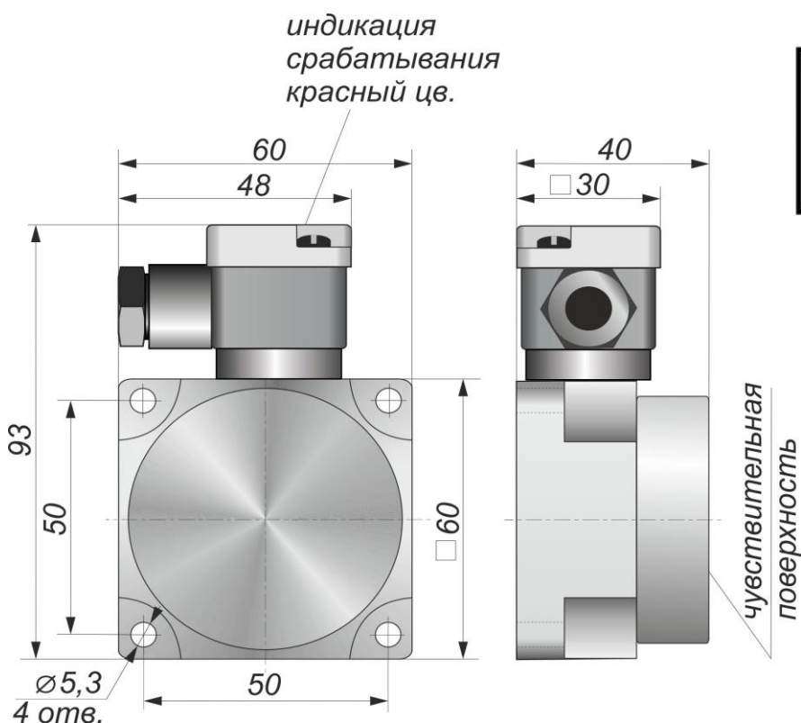
Габаритный чертеж
