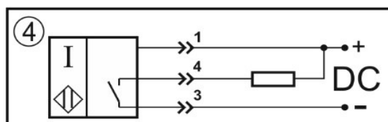
Цоколевка разъема
