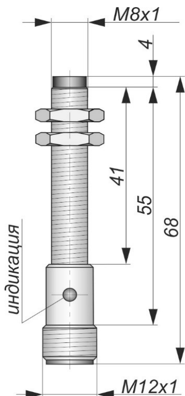
Габаритный чертеж
