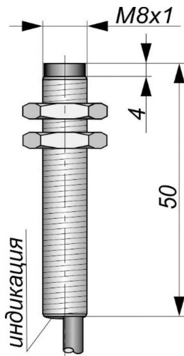
Габаритный чертеж
