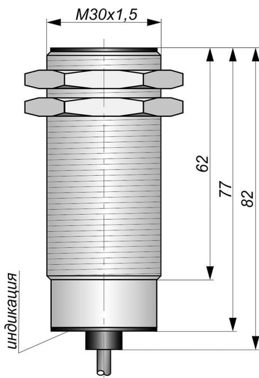
Габаритный чертеж
