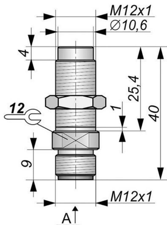
Габаритный чертеж
