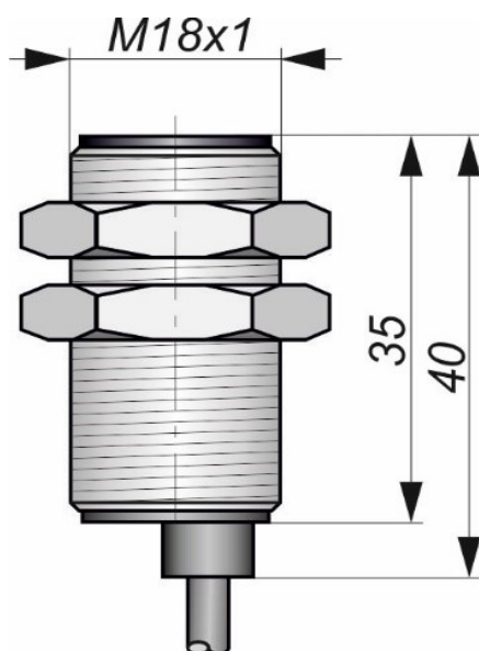
Габаритный чертеж
