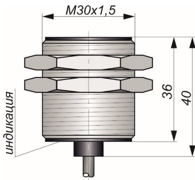
Габаритный чертеж
