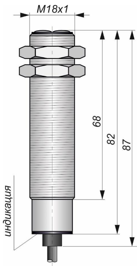
Габаритный чертеж
